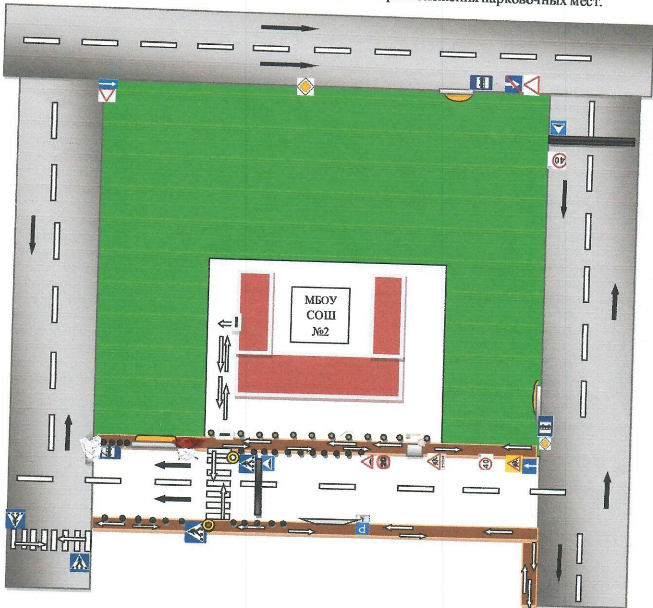
Схема организации дорожного движения в непосредственной близости от МБОУ СОШ №2 с размещением соответствующих технических средств организации дорожного движения, маршруты движения детей и расположения парковочных мест.
